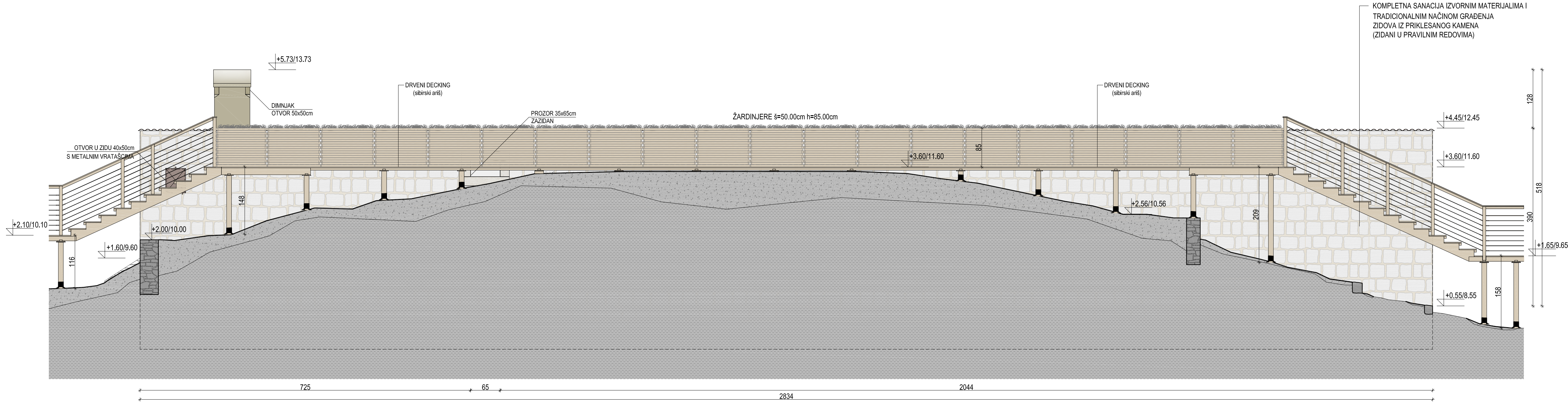
JUGO-ZAPADNO PROČELJE
